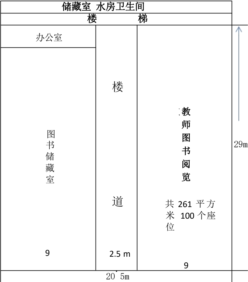
玉田职教中心电子商务专业图书馆建筑面积平面图
